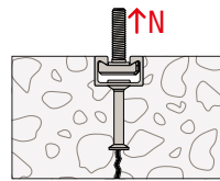
Betonversagen Spalten
