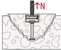
Kegelförmiger Betonausbruch
