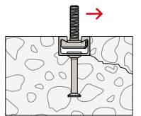
Betonkantenbruch
