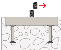
Stahlversagen Hammerkopfschraube ohne Hebelarm
