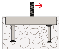
Stahlversagen zwischen Anker und Schiene
