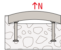
Stahlversagen Biegung der Schiene
