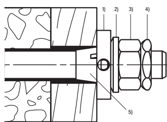
Durchsteckmontage mit FIS A und Injektionssystem FIS SB Größen: M12, M16, M20, M24
