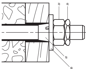
Durchsteckmontage mit FIS A und Injektionssystem FIS SB Größen: M20, M24
