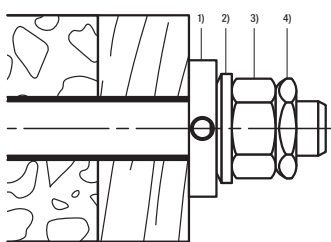
Vorsteckmontage mit FIS A und Injektionssystem FIS SB Größen: M12, M16, M20, M24
